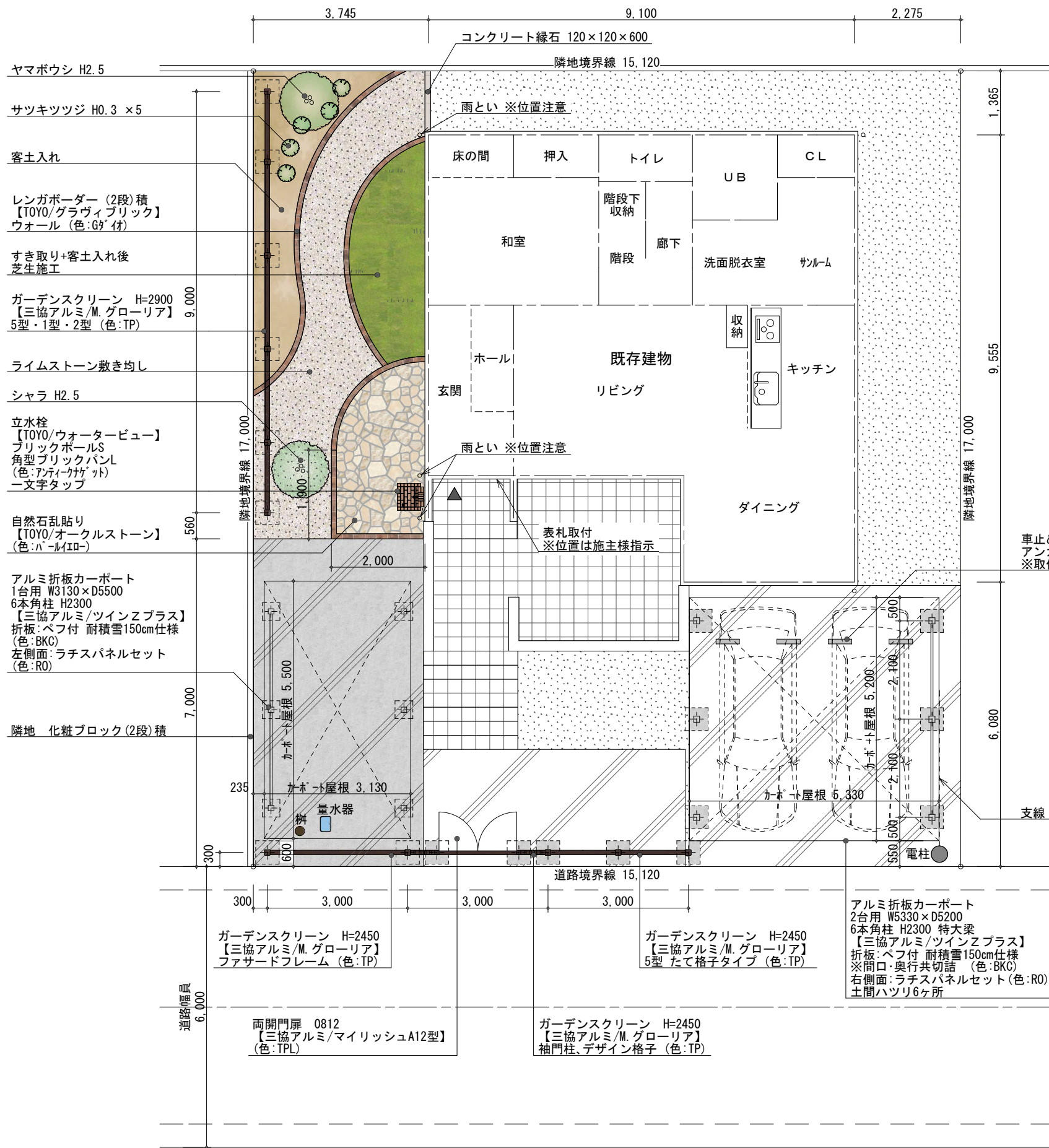
平面図 S:1/100
