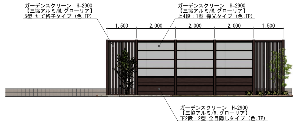
立面図 S:1/100
